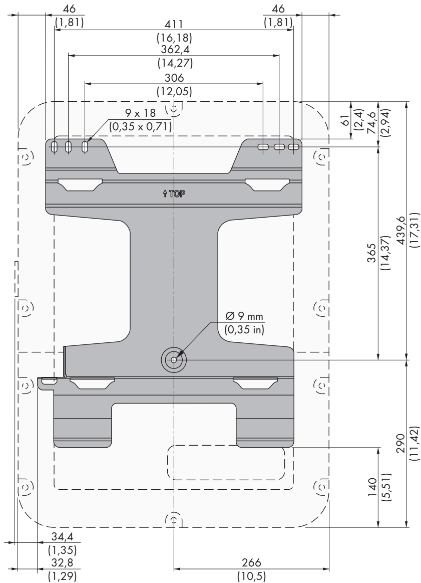
Figure 3 : Position des points de fixation (Dimensions en mm (in))
