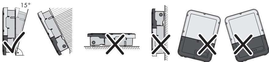
Figure 5 : Positions de montage autorisées et non autorisées
