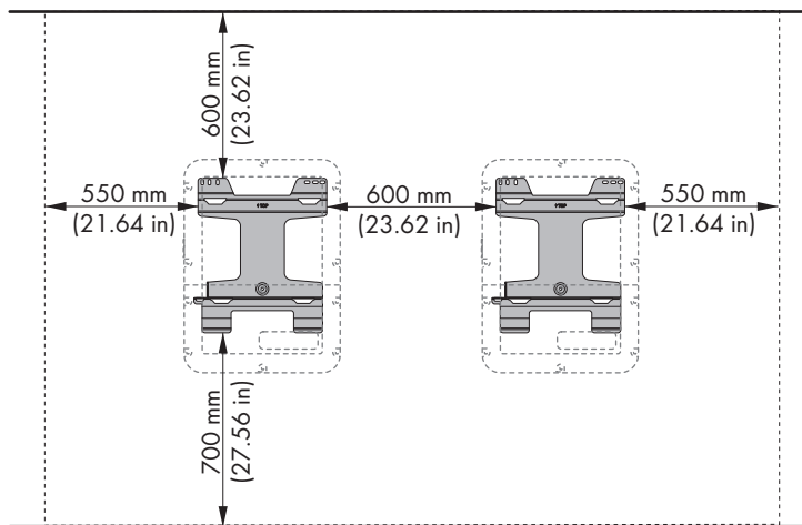
Figure 4 : Distances recommandées (Dimensions en mm (in))
