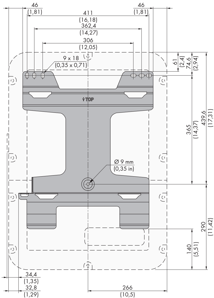
Imagen 3 : Posición de los puntos de fijación (Medidas en mm (in))
