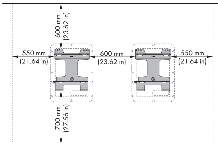
Imagen 4 : Distancias recomendadas (Medidas en mm (in))
