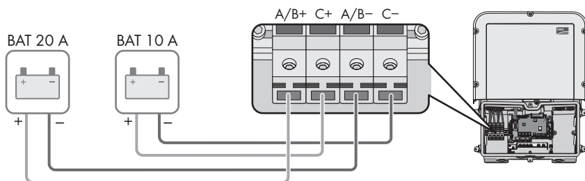
Imagen 9 : Tipos de conexión (ejemplo)
