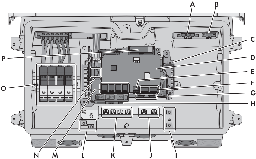
Imagen 8 : Áreas de conexión del interior del inversor
