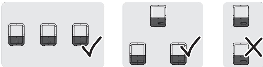
Figure 6 : Positions de montage autorisées et non autorisées de plusieurs onduleurs
