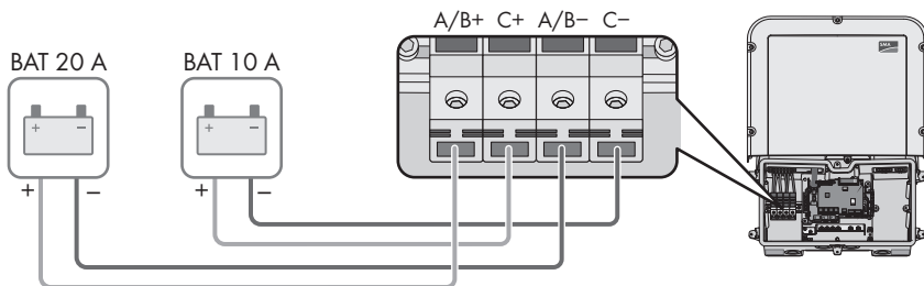
Figure 9 : Possibilités de raccordement (exemple)
